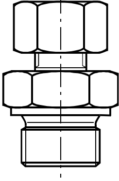
Klemmverschraubung mit abgesetztem Dichtbund
