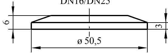
Blindflansch nach DIN32676 DN16/DN25
