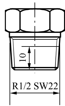
Verschraubung mit kegeligem Gewinde Bsp. R1/2
