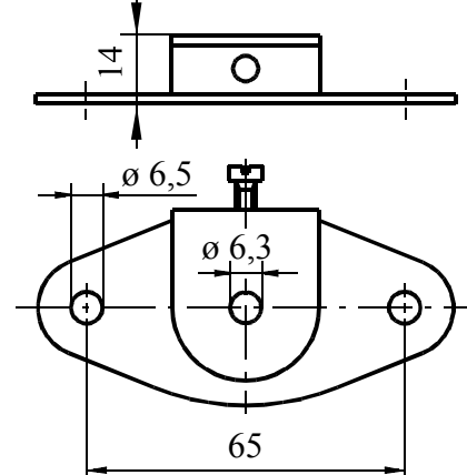
Blechflansch Stahlblech verzinkt
