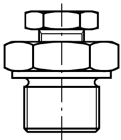
Klemmverschraubung totraumfrei
